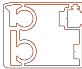
TELAIO ANTA VETRO SINGOLO SINGLE GLASS SHUTTER FRAME 16.162
