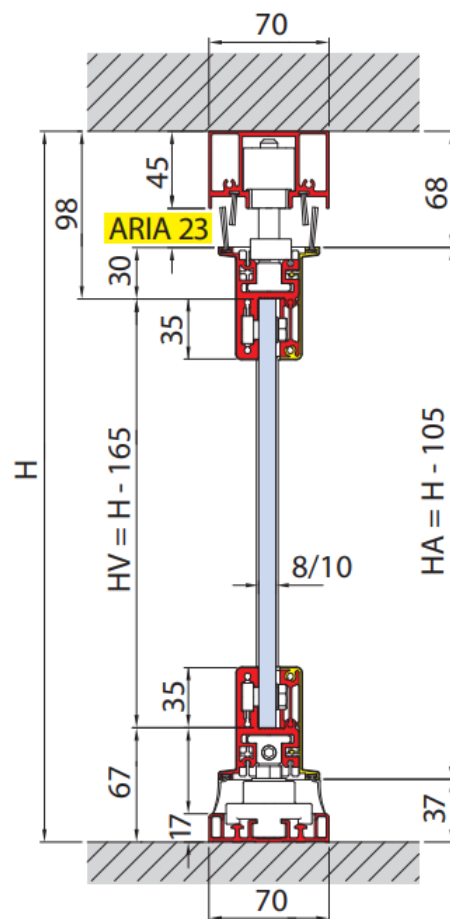
DETTAGLIO SEZIONE VERTICALE
