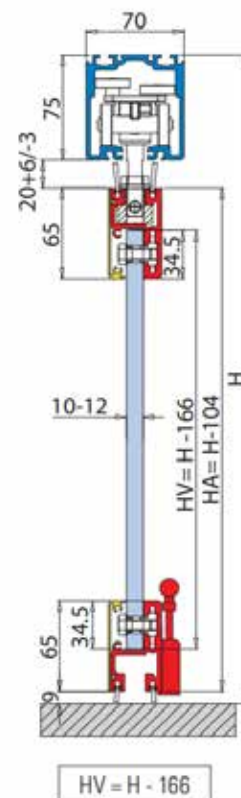
DETTAGLIO SEZIONE VERTICALE
