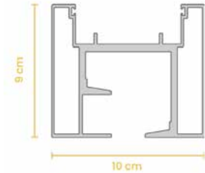
DETTAGLI BINARIO
